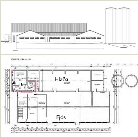
Teikningar: Stöð verkfræðisstofa ehf. Fjósíð á Hólum. Aðalteikning. Ljósmyndir: Anna Björg Bjarnadóttir, 2023
